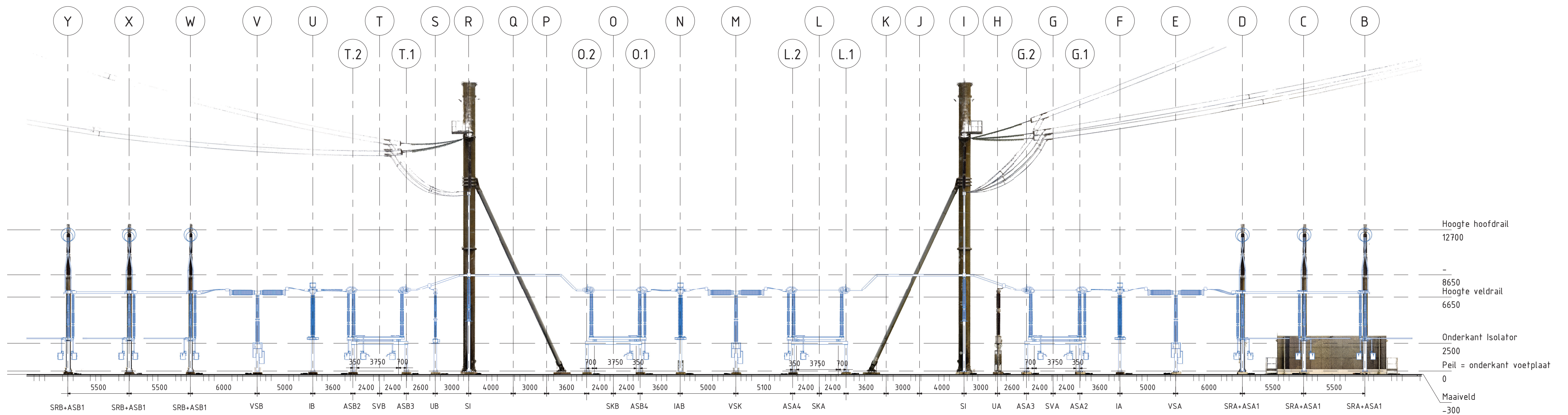
2 Zijaanzicht Schaal 1 : 200
